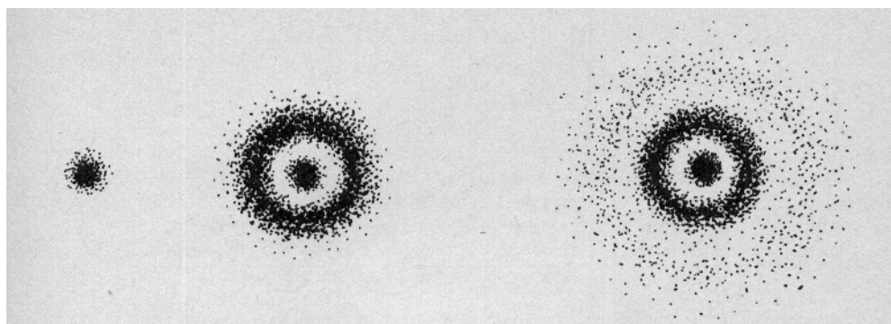
Densidad electrónica en un plano de corte transversal para electrones 1s, 2s y 3s, átomo de hidrógeno (The Principles of Inorganic Chemistry, W., L., Jolly)
